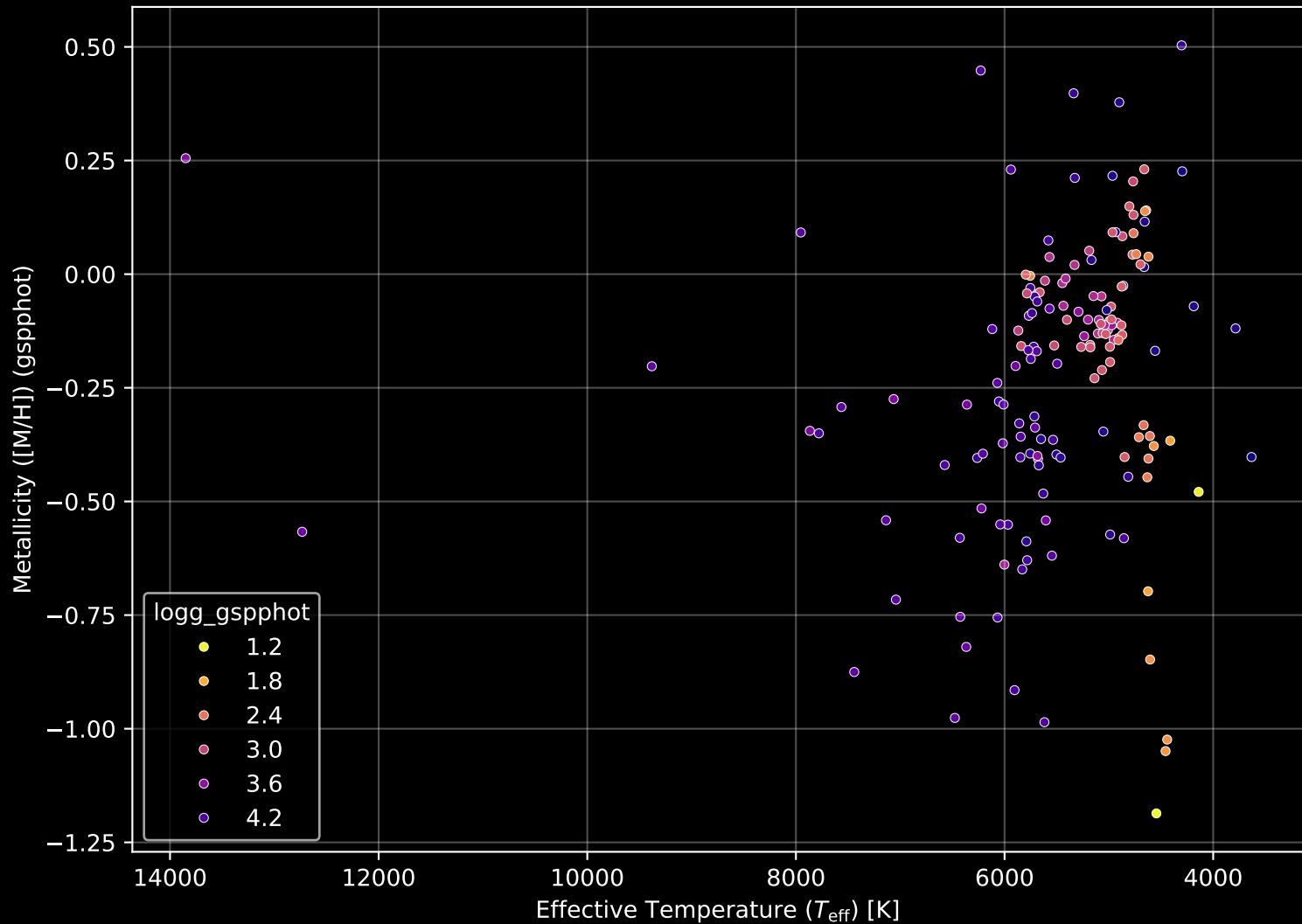
APOGEE DR17 Field: [270-20-O] Stellar Population Parameters (n= 158)
